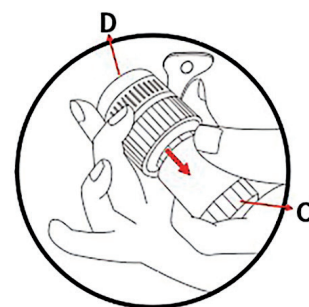
Demontaż - kombinacja C+D Disassembly diagram The combination of C + D
